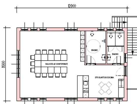
PRIMO PIANO
